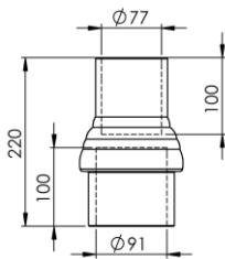
REDUSER Ø90 - Ø 76
