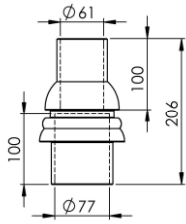
REDUSER Ø76 - Ø 60
